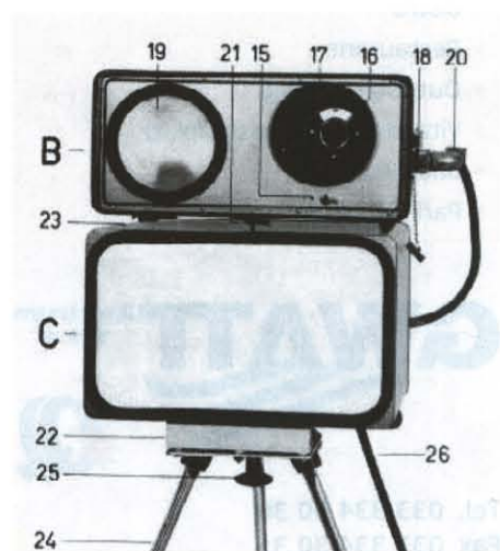
MU 58-44 (mobiles Radarmessgerät aus den 50er Jahren)
